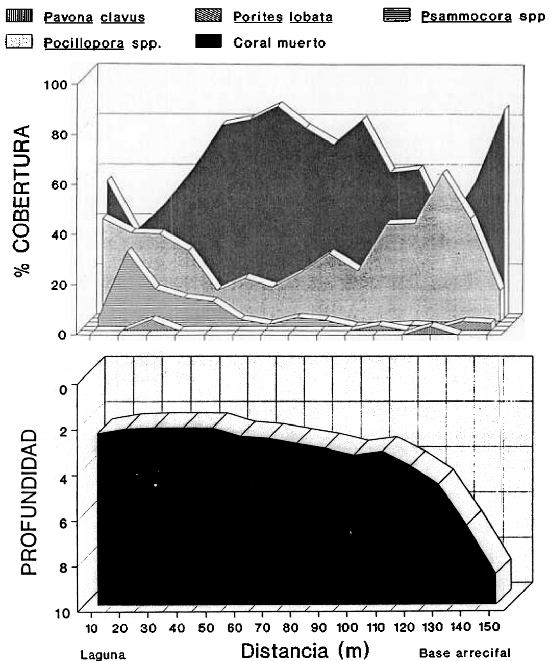
Fig. 2. Perfil sinóptico de zonación y cobertura de corales escleractíneos (A) y profundidad durante la marea alta (B), del arrecife de Isla Iguana, para agosto de 1988. Basado en los datos de los transectos # 4-7 y 18-21.
